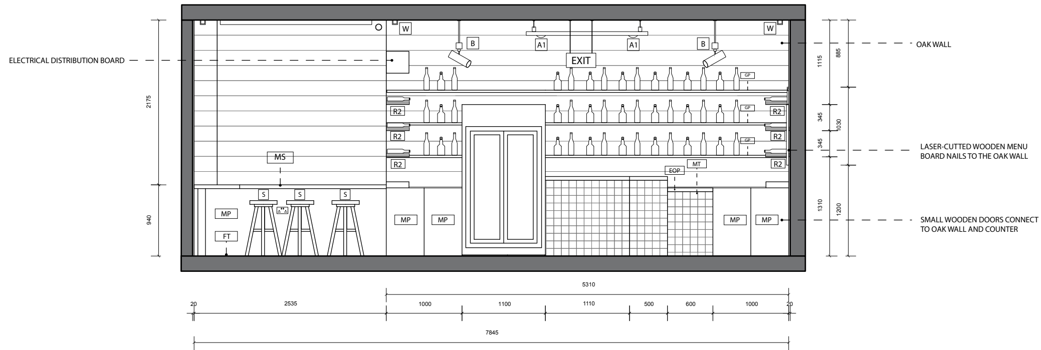
A A202 ELEVATION A 1:50
