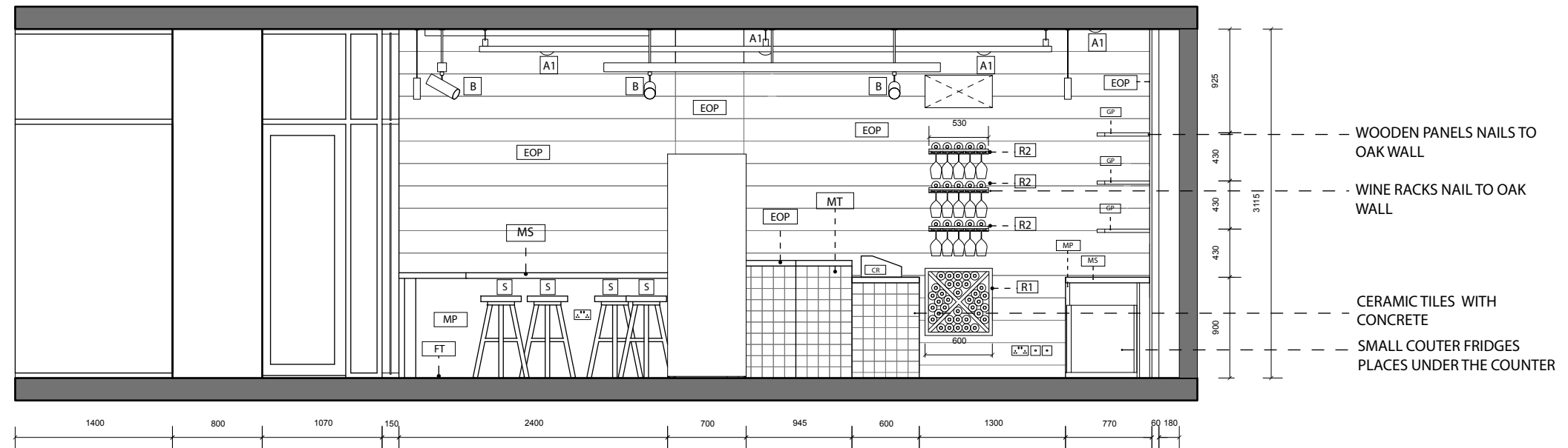
A SECTION A A201 1:50
