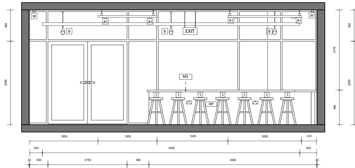
B A202 ELEVATION B 1:50
