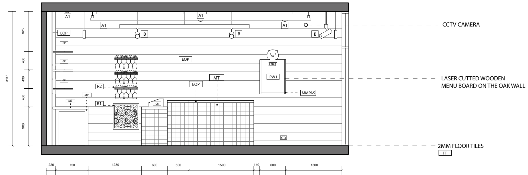
B SECTION B A201 1:50
